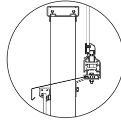
Alakiskon kiinnitys ja vedenohjaus tapahtuu hallitusti vesipellin avulla.
