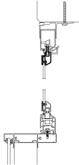
Alutec 3 pystyleikkaus parvekelasituksenä
